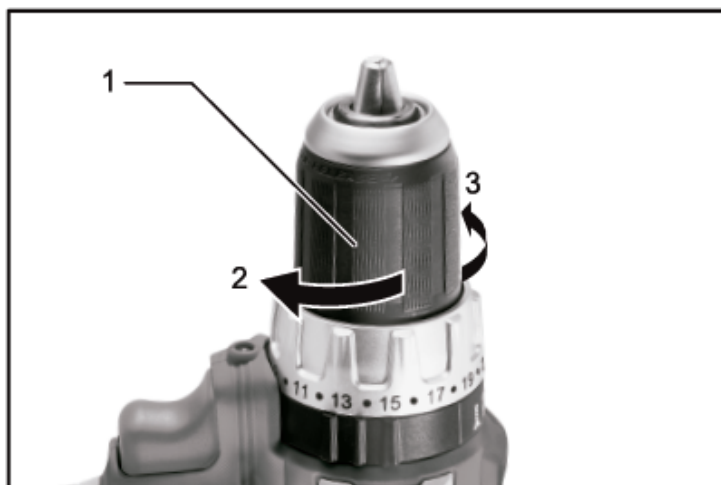
1. Mandril 2. Fechar 3. Abrir
